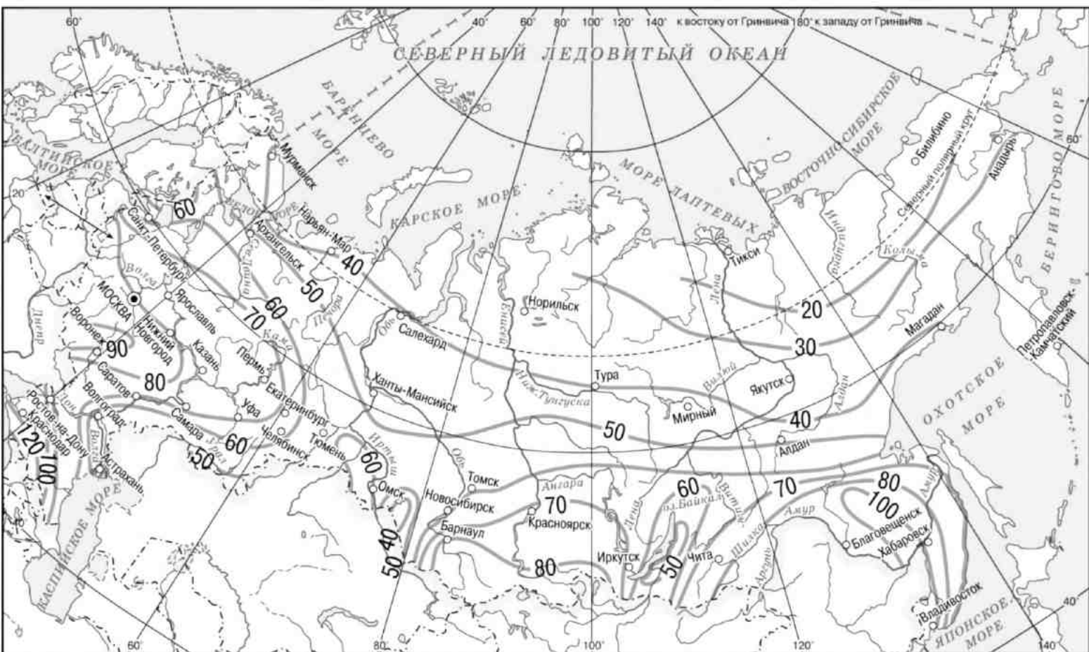
Рисунок Б.1 – Значения величин интенсивности дождя q_{20}
